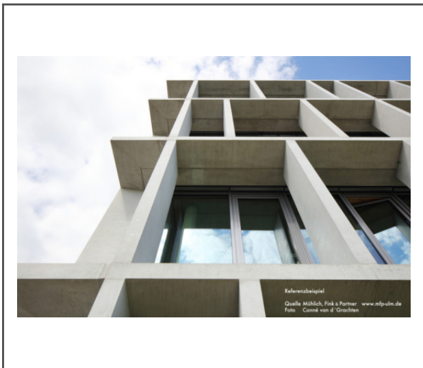
Fassade Detail
